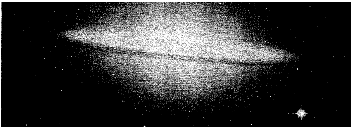
Una galassia spettacolare fotografata dal telescopio spaziale Hubble.
