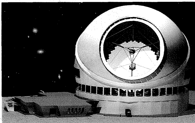
Dall'alto, un'altra visione stellare catturata da Hubble; come sarà l'Elt, European extremely large telescope.
